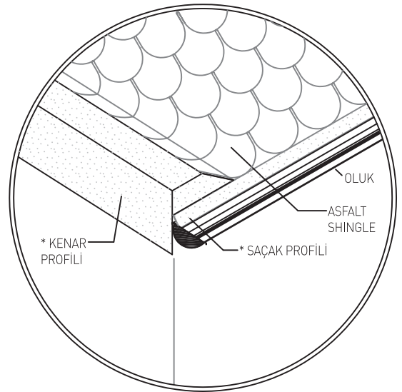
B DETAYI
